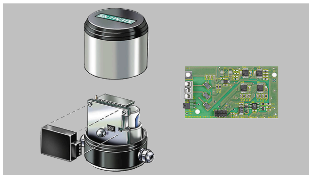
Modbus/Encoder module
